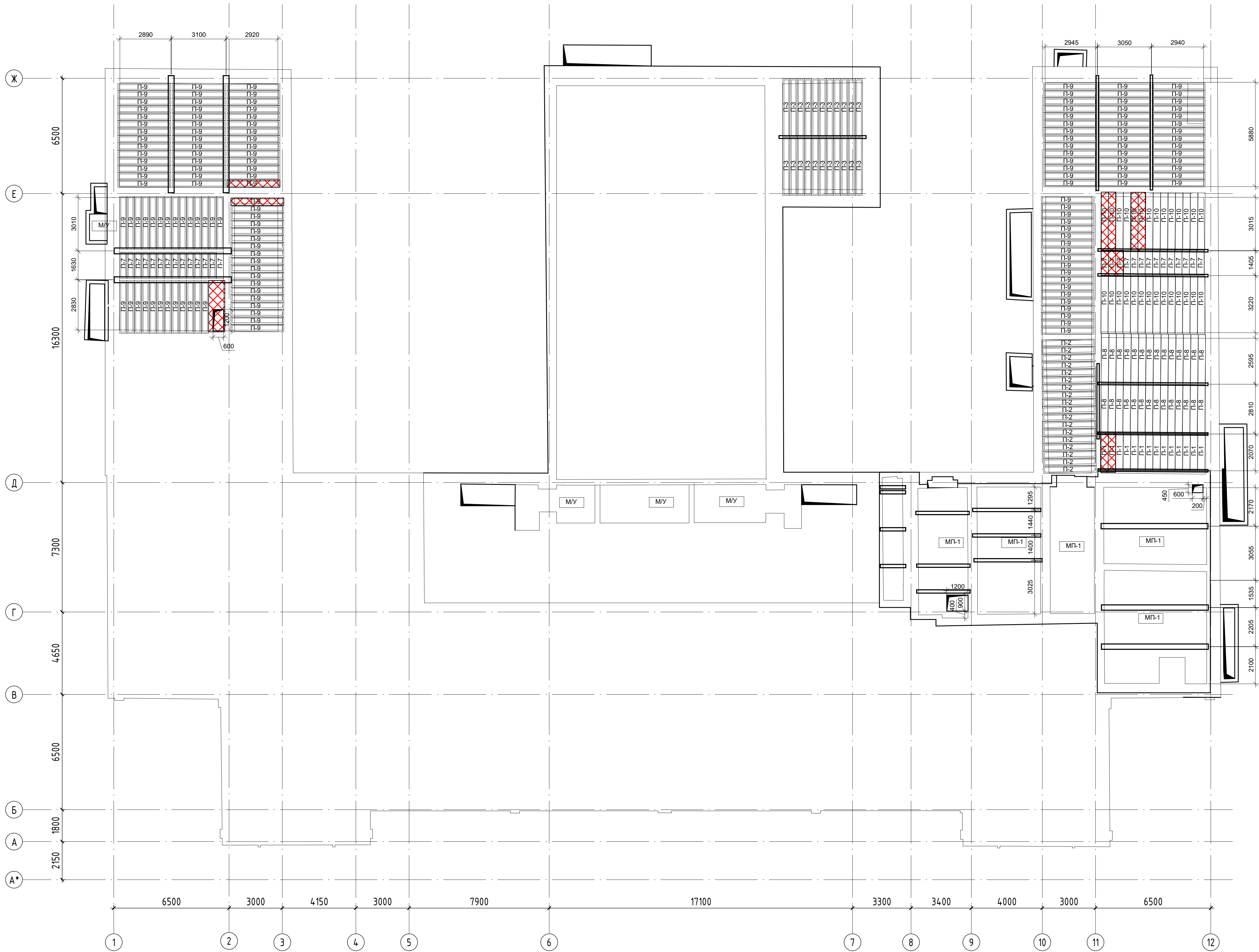
Схема перекрытия над подвалом с указанием заменяемых плит и монолитных участков (1 : 100)
